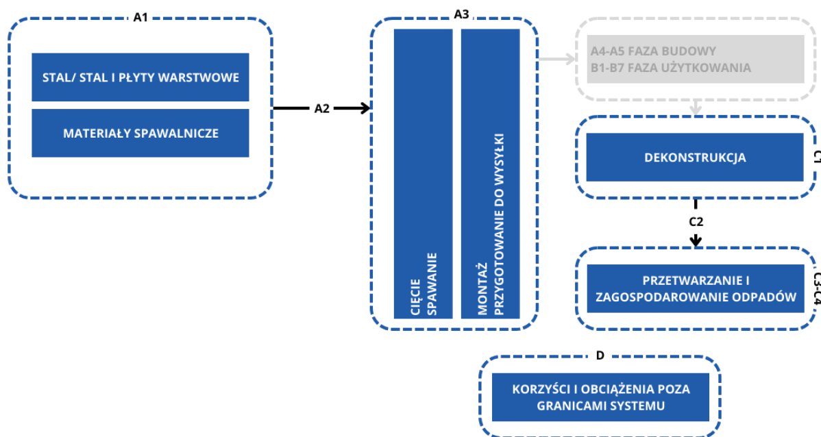
Rysunek 5.1: Granice systemu dla charakterystyki środowiskowej
